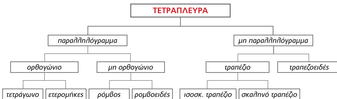
Διάγραμμα 3: Η ταξινόμηση των τετραπλεύρων κατά τον Ποσειδώνιο και τον Ήρωνα
